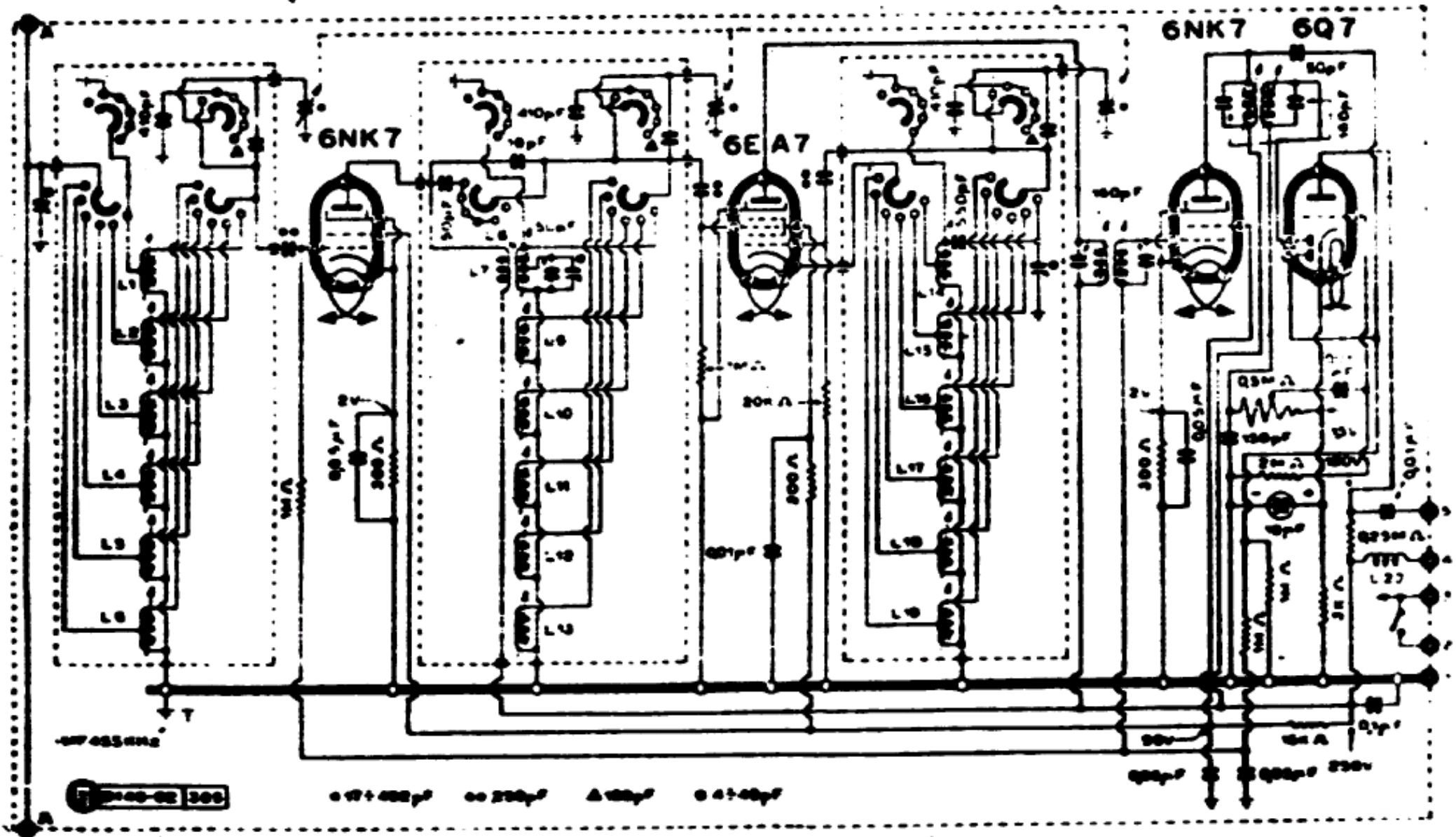
L.R.I. AUTOVOX - MODD. « RA2/C6 » « RA2/C12 » PARTE AF - MF - RIV.
